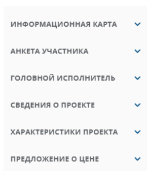
Рисунок 5 - Панель навигации
